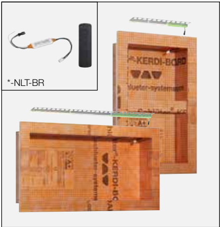
Kit Schlüter®-KERDI-BOARD-NLT pour réalisation de niches avec effets lumineux
