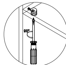
Schemat złącza mimośrodowego
