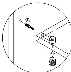
Schemat złącza mimośrodowego
