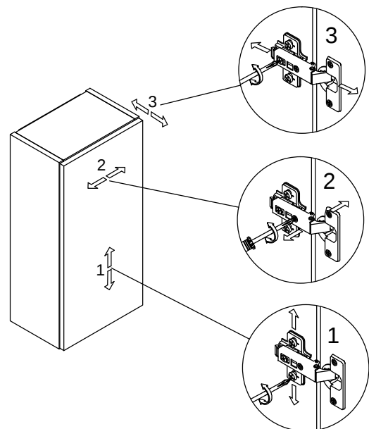
Rys.4. Regulacja ustawień drzwiczek.
