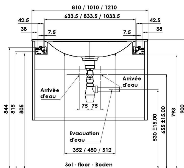
Montage en option avec trop plein invisible vasque solid surface. BONDE INNOVA Réf. 707004000050 Installation with optional invisible overflow Option : BONDE INNOVA Réf. 707004000050 Montage mit Clou-System als Option : BONDE INNOVA Réf. 707004000050
