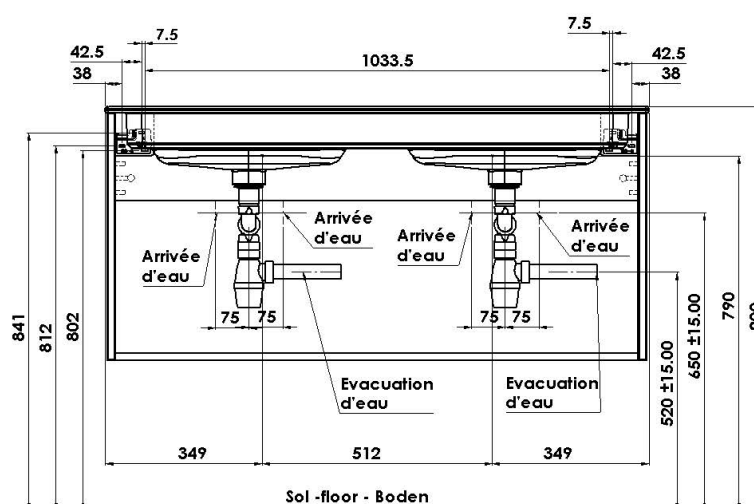
Montage vasque ceramique Installation ceramic Montage Keramik
