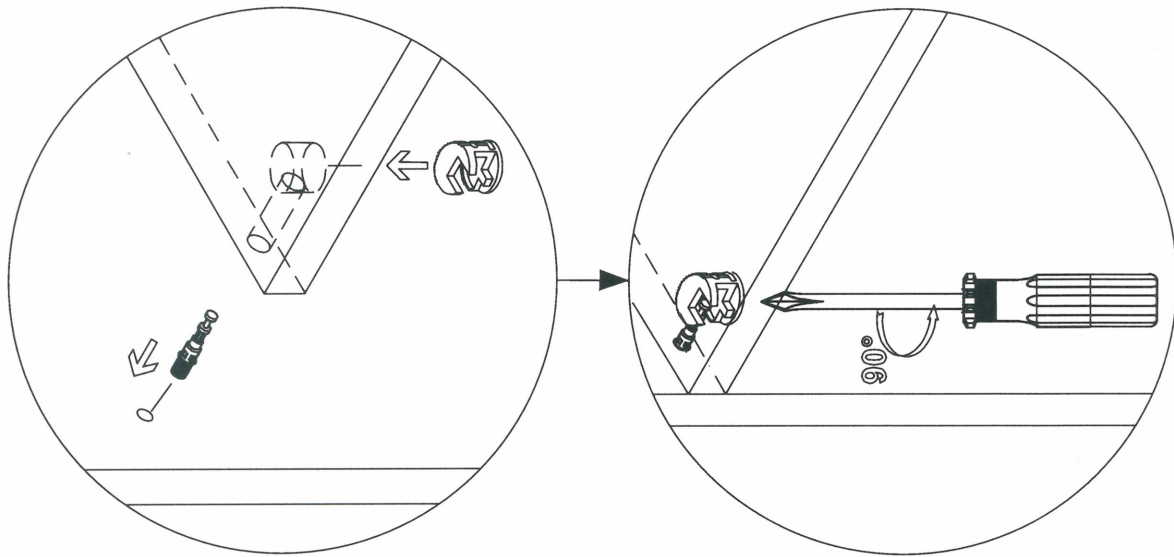
Rys. 1 Schemat złącza mimośrodowego
