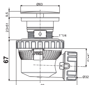
NANO 6.7 écoulement libre
