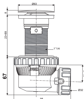
NANO 6.7 bonde 100 mm
